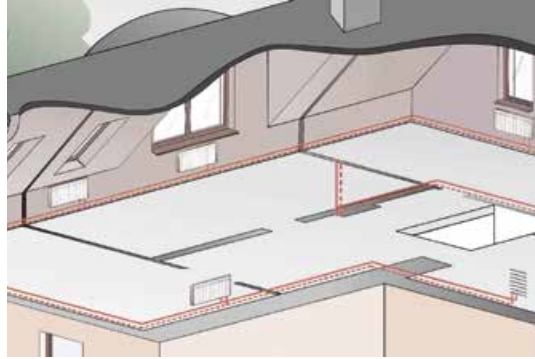
Sustav petlje u dvocijevnoj instalaciji grijanja
